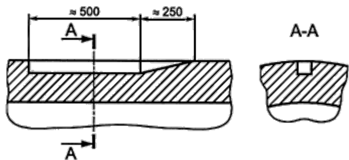
Рисунок 6 - Канавка, обрабатываемая на наружной поверхности трубы
