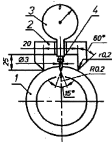
1 - труба; 2 - специальная призма ( \angle = 30 ); 3 - индикатор ИЧ-02 ГОСТ 577; 4 - специальный наконечник
